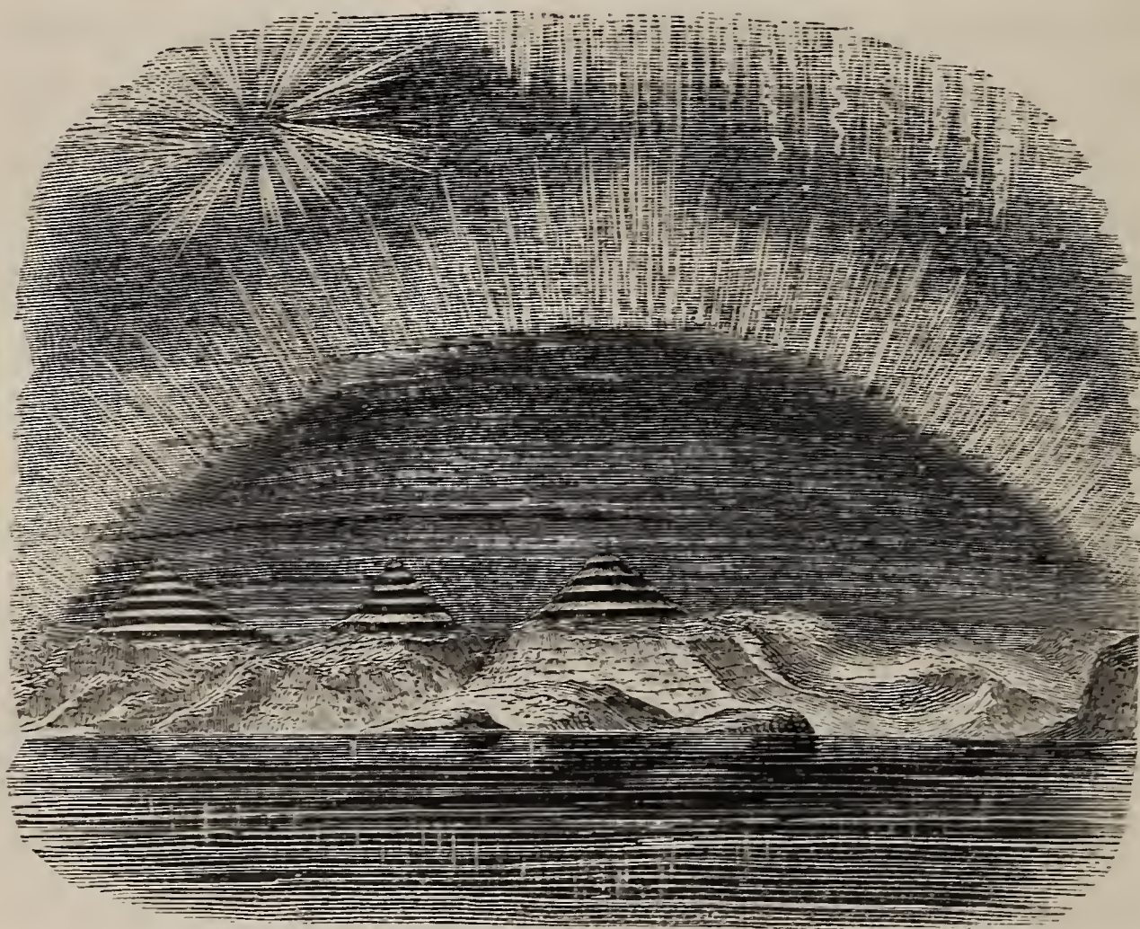
AURORA BOREALIS.
